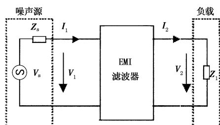
V_s 为噪声源, Z_s 为噪声源阻抗, Z_1 为噪声的负载阻抗
