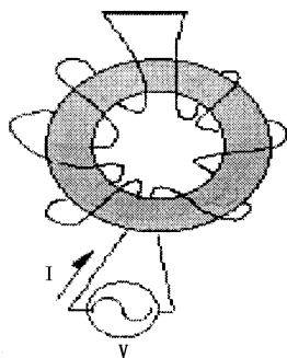
图5 共模电感的漏感测量
