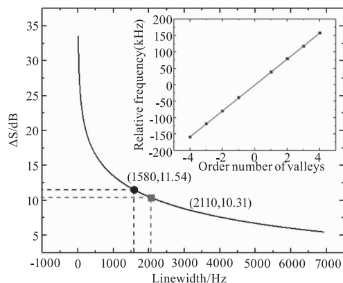
图6 估计激光线宽的CDSPT对线宽的依赖性
